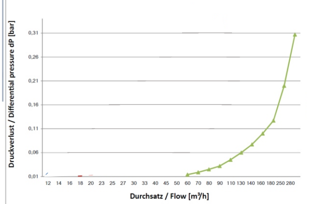
Flanschfilter DN 150 100µm
