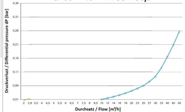
Flanschfilter DN 65 100µm
