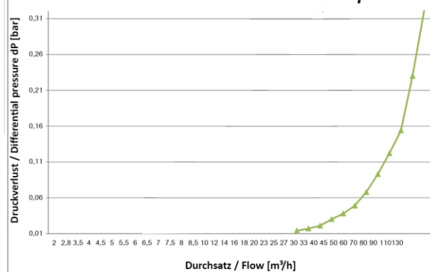
Flanschfilter DN 100 100µm
