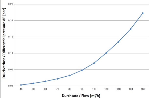
Flanschfilter DN 125 100µm
