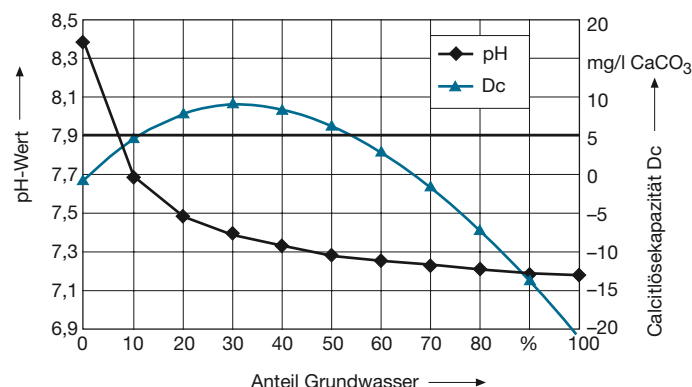
BILD 1 PH-WERT UND CALCITLÖSEKAPAZITÄT DC eines Mischwassers aus Fernwasser und hartem Grundwasser
