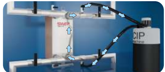
Spülen Sie den Wärmetauscher, indem Sie Wasser über den unteren Anschlusspunkt einfüllen. Spülen Sie solange, bis das Wasser neutral ist (pH 7).
